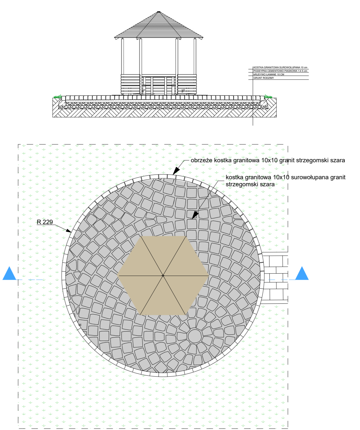
detal D-2 przekrój a-a
