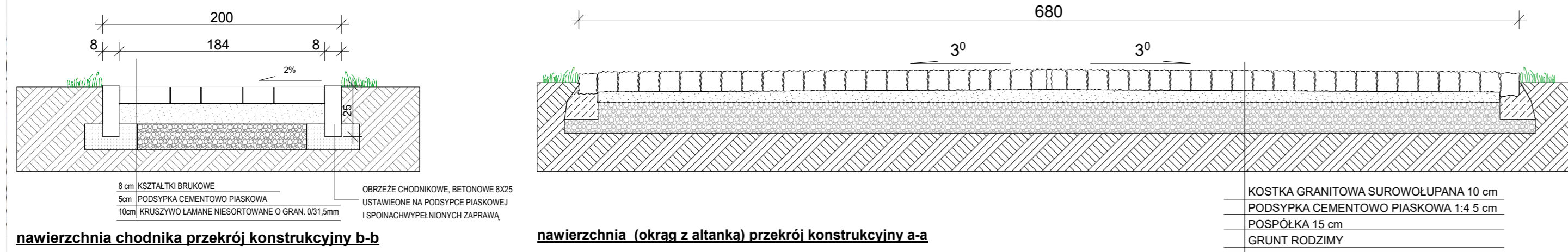
nawierzchnia chodnika przekrój konstrukcyjny b-b
