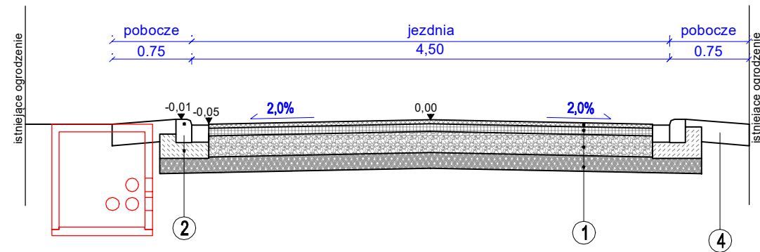
PRZEKRÓJ KONSTRUKCYJNY droga publiczna
