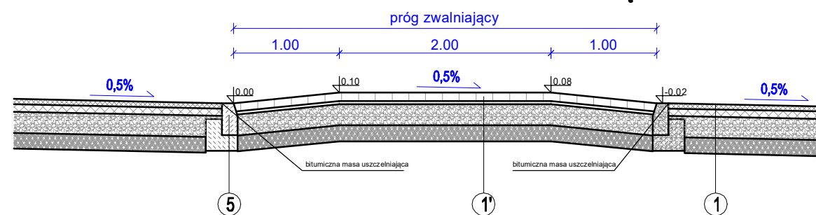
PRZEKRÓJ PODŁUŻNY PROGU ZWALNIAJĄCEGO
