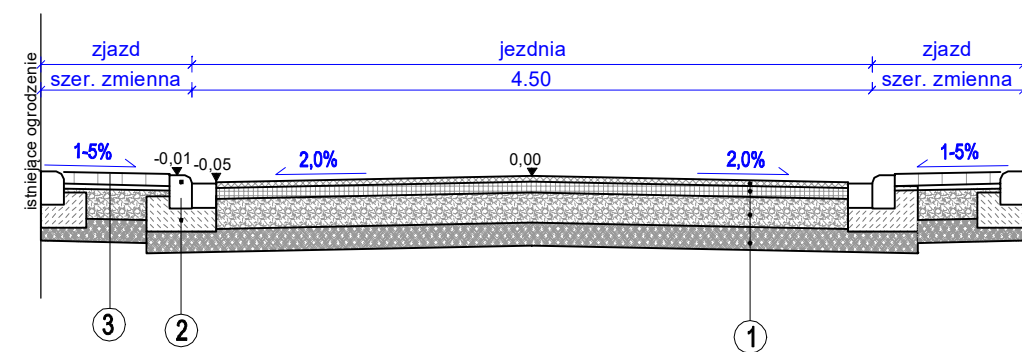
PRZEKRÓJ KONSTRUKCYJNY droga publiczna w miejscu zjazdów
