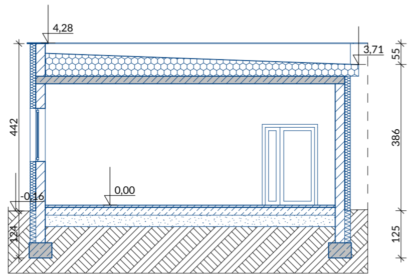
PRZKRÓJ B-B
