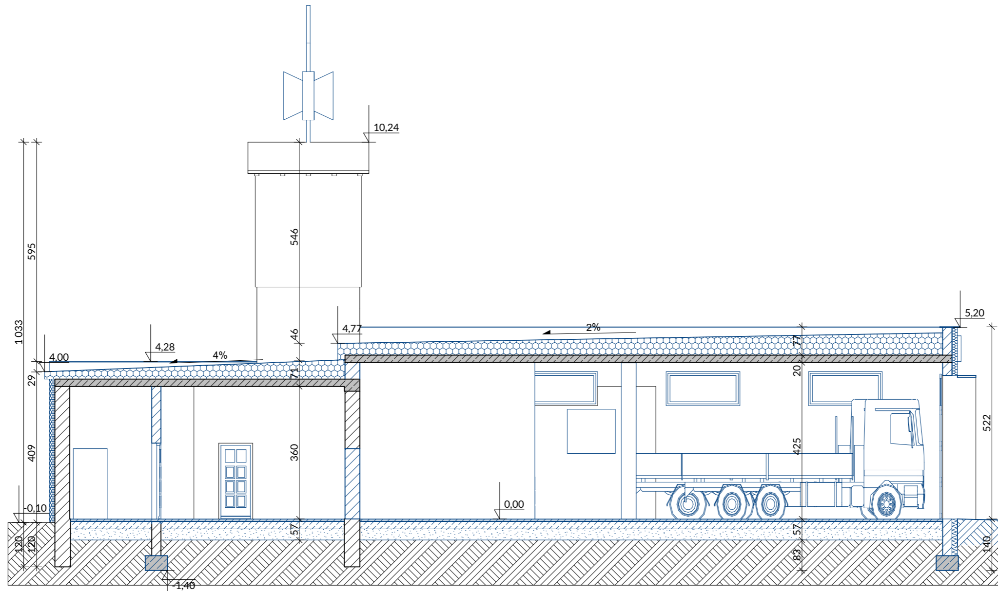
PRZKRÓJ A-A
