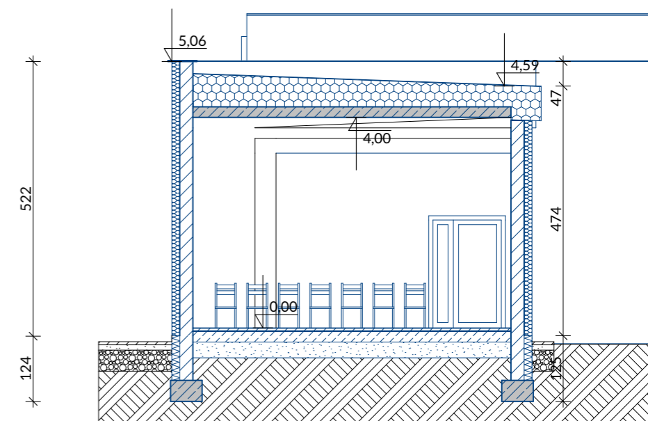
PRZKRÓJ B-B
