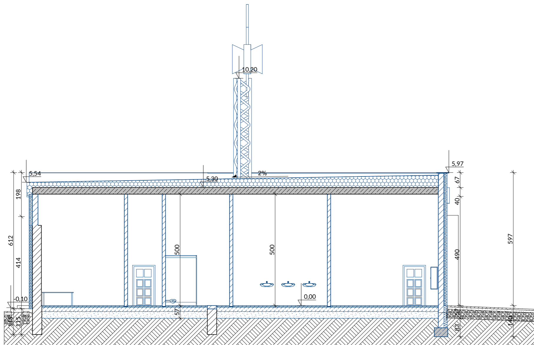
PRZKRÓJ A-A
