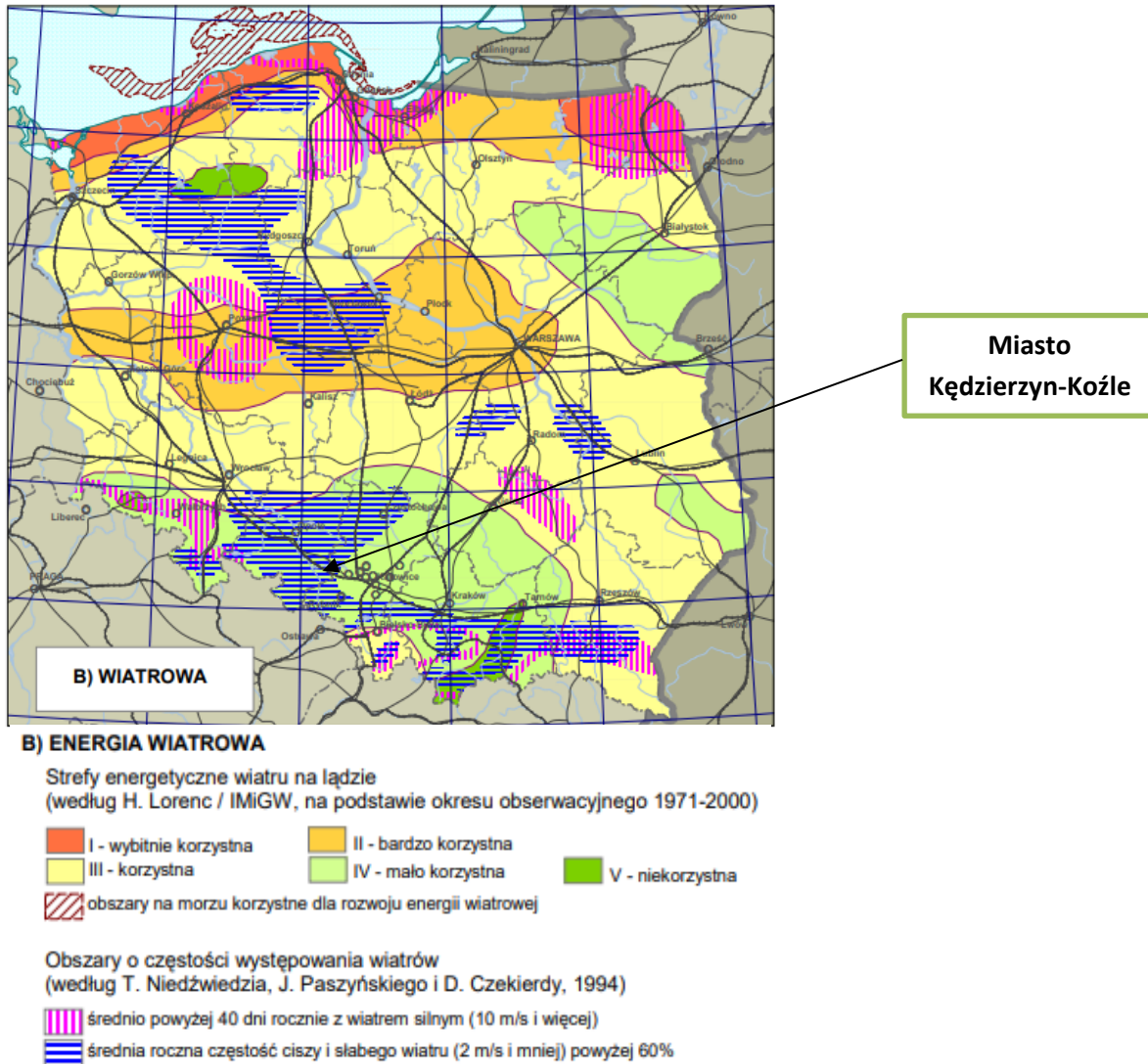
Rysunek 6. Strefy energetyczne wiatru na łądzie (według H. Lorenc/IMI GW, na podstawie okresu obserwacyjnego 1971-2000)
