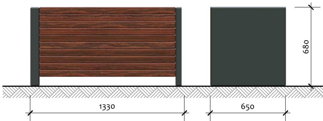
WIDOKI Z BOKU
