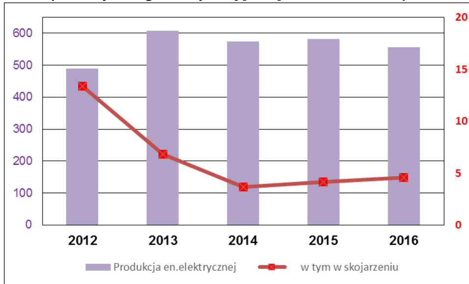
Wykres 5-1 Roczna produkcja energii elektrycznej [GWh] w TAMEH Polska sp. z o.o. ZW Błachownia
